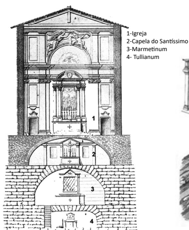
Figura 14. Corte da Igreja de Giuseppe dei Falegnami , Roma.
