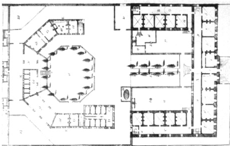
Figura 37. Planta Walnut Street Prison , Filadélfia, Pensilvânia, 1775.
