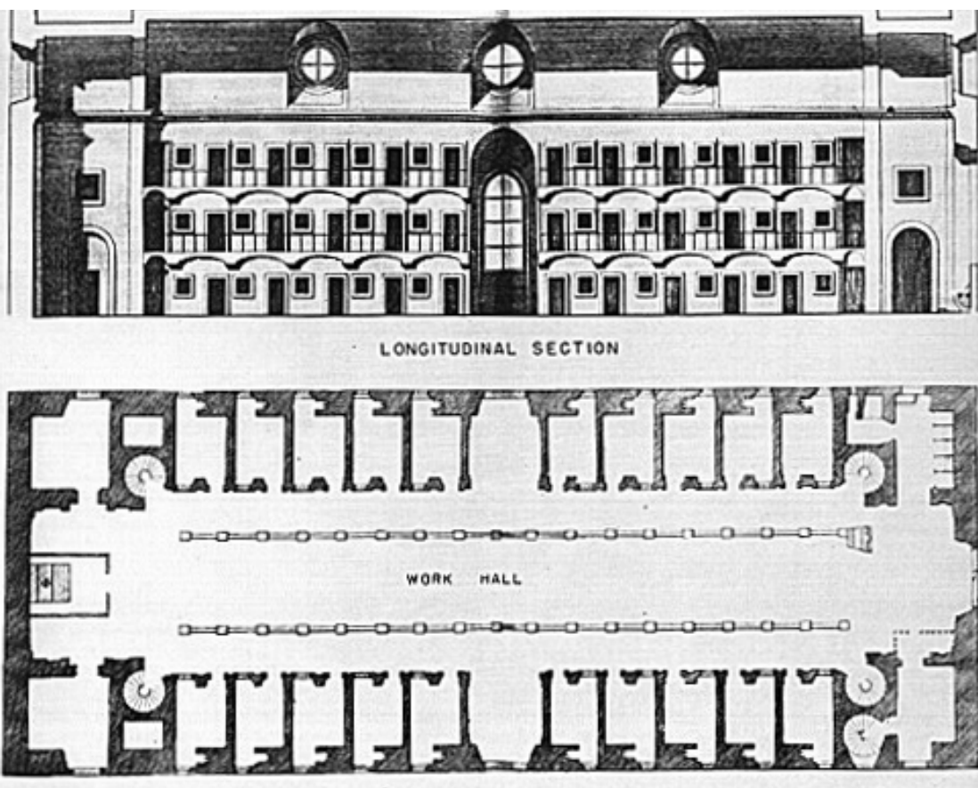
Figura 28. Vista, corte e planta da Casa de Correção de San Michele , arquiteto Ferdinando Fuga, Roma, 1704.
