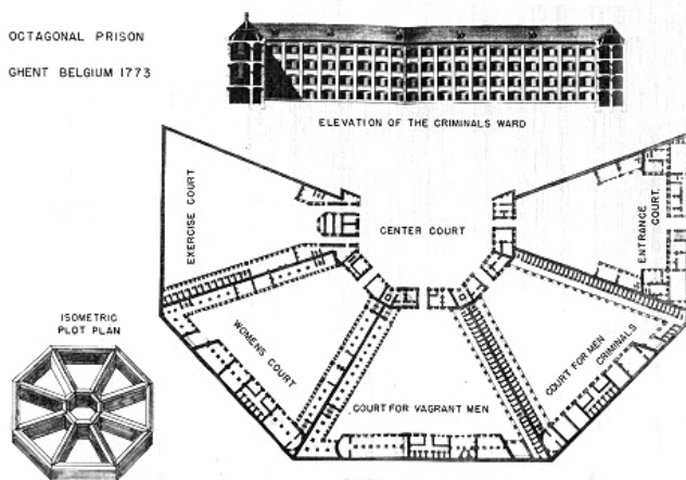
Figura 30. Planta da Casa de Detenção Maison de Force , próximo a Ghent, 1772-1775.
