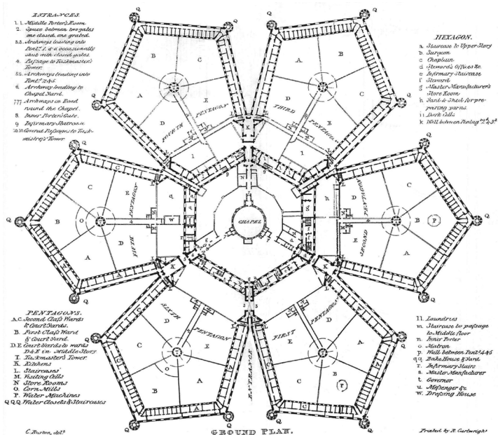
Figura 34. Planta da Millbank Penitentiary , 1812.
