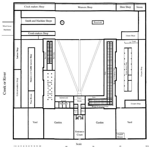
Figura 46. Planta da Auburn State Prison , Nova Iorque, 1816.
